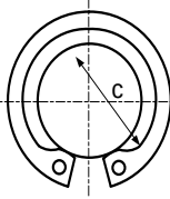
حلقة مرنة للأجواف NF E 22 -165
